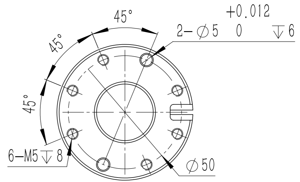
B向 连接法兰尺寸
