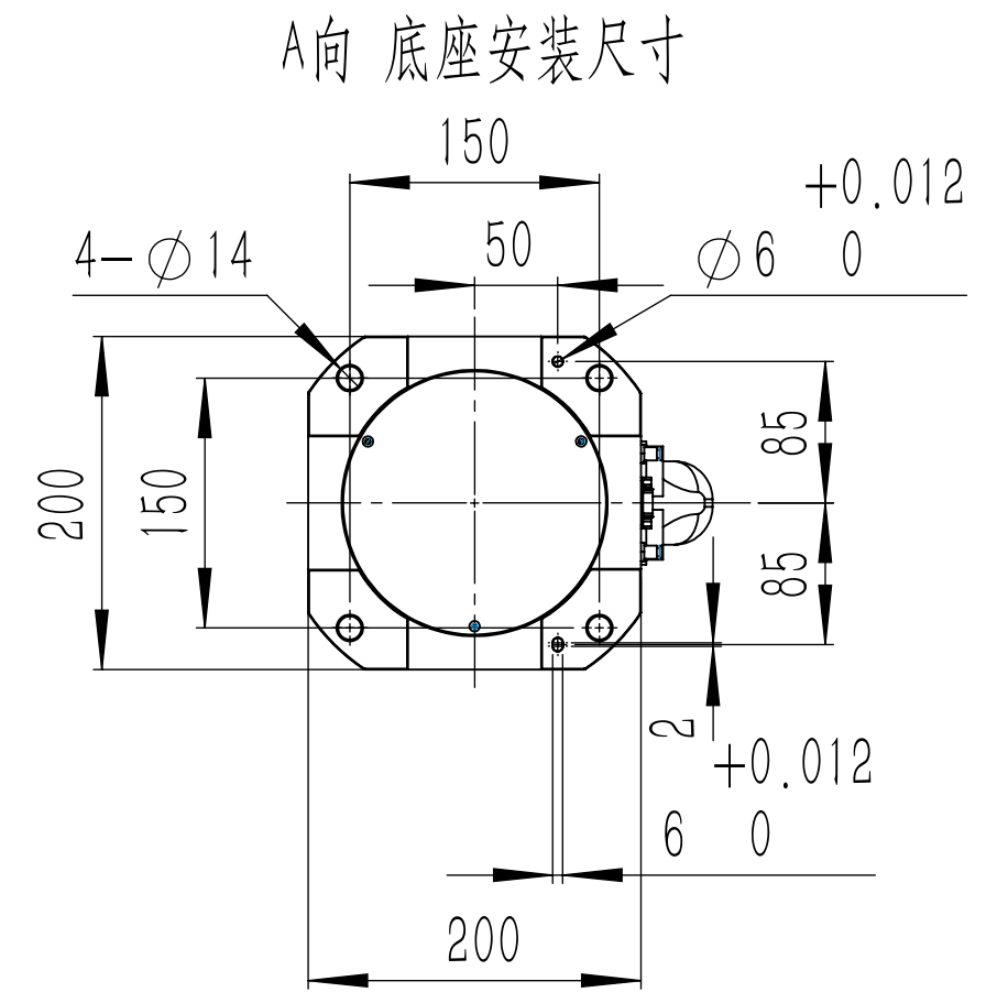
C4-0605外形尺寸图
