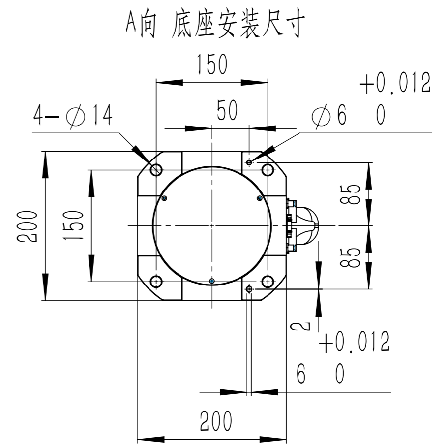
C4-0605F外形尺寸图
