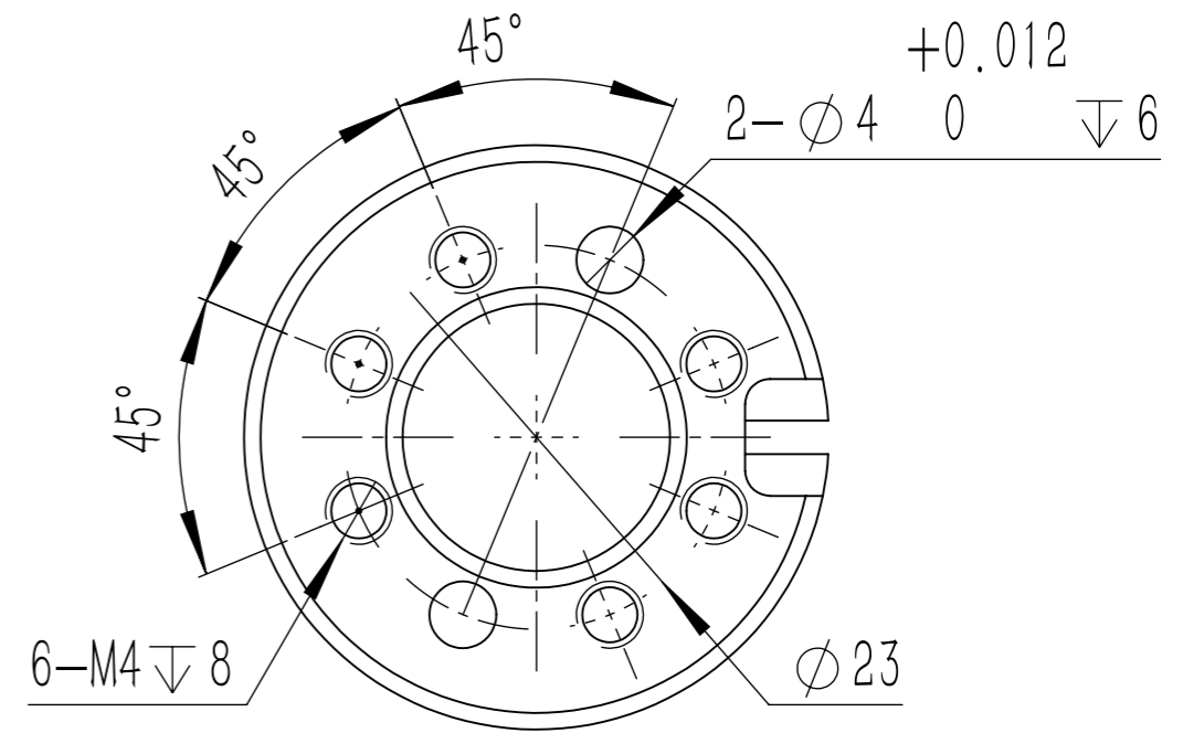
B向 连接法兰尺寸
