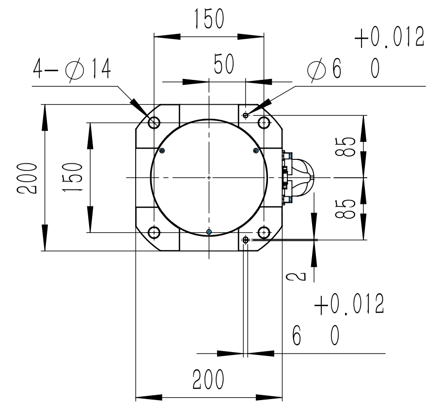
A向 底座安装尺寸
