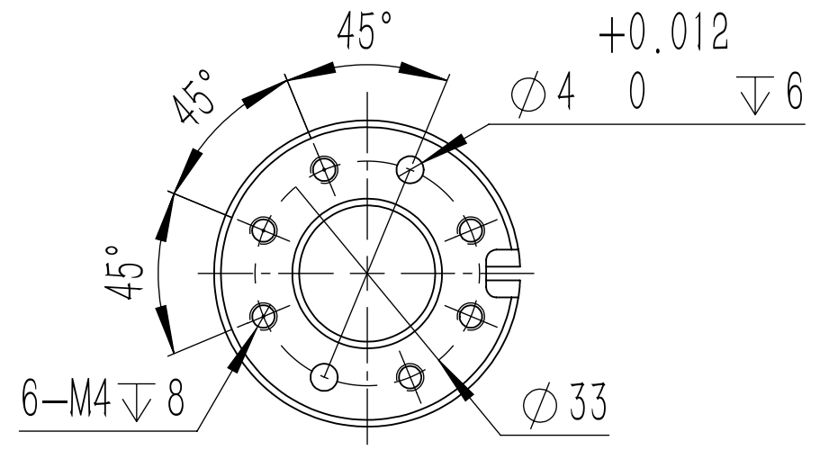
B向 连接法兰尺寸
